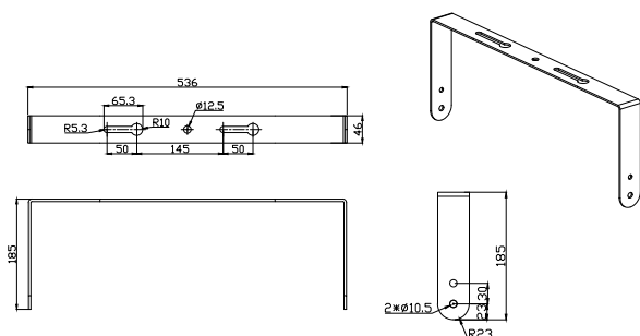
1,2 模組 单位:mm
