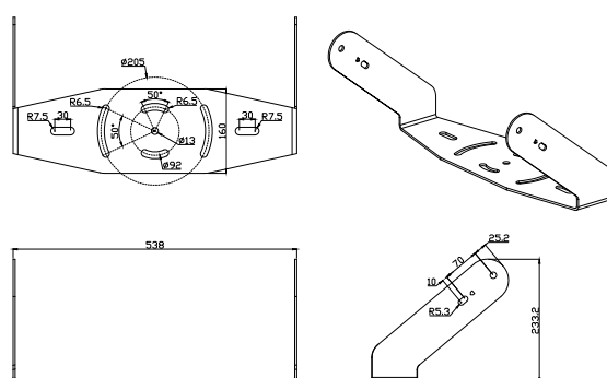
3模组 单位:mm
